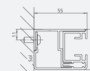
Montage intrados
