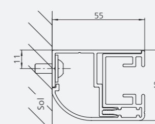
Montage intrados
