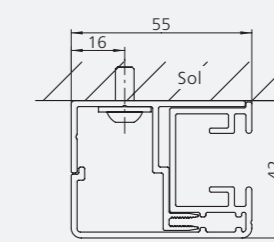
Montage mural
